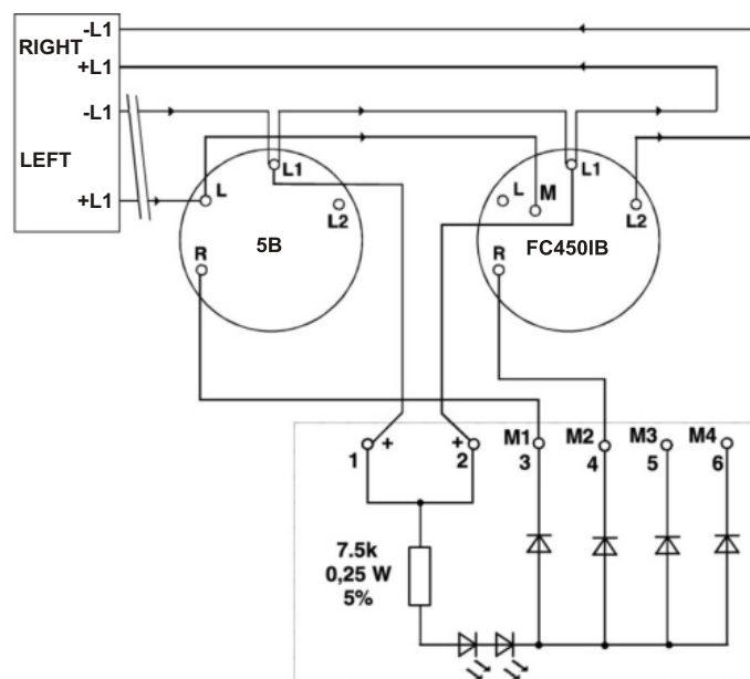
FIG. 2 Schema di collegamento del 801HL
