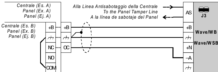
Fig. 3 - Ⓐ Esempio di collegamento per attivare la sirena Wave/WB o Wave/WSB tramite il morsetto -A Ⓑ Connection using Terminal -A to activate Wave/WB or Wave/WSB Ⓒ Ejemplo de conexión para activar la sirena Wave/WB o Wave/WSB mediante el borne -A
