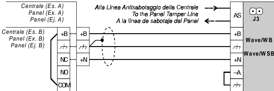
Fig. 2 - Ⓐ Esempio di collegamento per attivare la sirena Wave/WB o Wave/WSB tramite il morsetto +N Ⓑ Connection using Terminal +N to activate Wave/WB or Wave/WSB Ⓒ Ejemplo de conexión para activar la sirena Wave/WB o Wave/WSB mediante el borne +N
