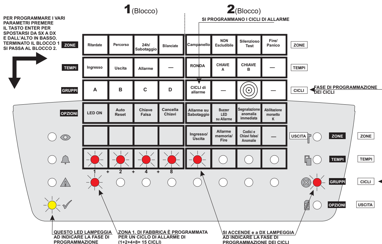
Figura 20 Schema di programmazione da tastiera dei Cicli.
