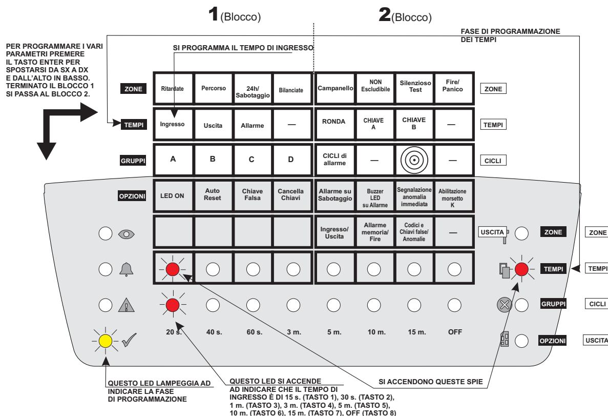
Figura 17 Schema di programmazione da tastiera dei Tempi.
