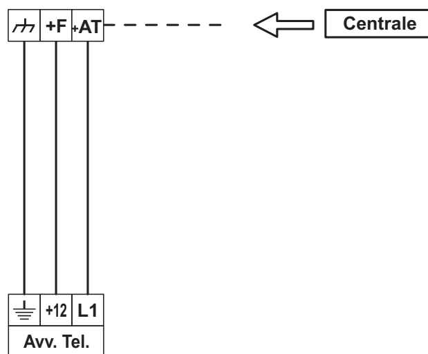
Figura 9 Collegamento dell'avvisatore telefonico.
